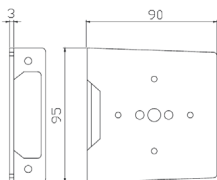
Equerre de fixation
