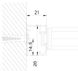
Coulisse pose tableau
