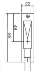
Dimensions platine renvoi cote intérieur
