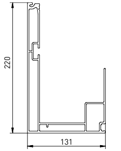
Dachrinne
