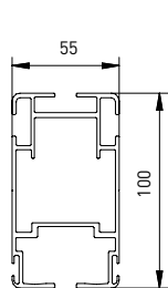
Führungsschiene
