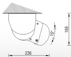
Pose plafond mini 15°
