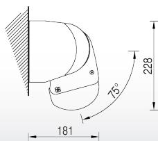
Pose de face maxi 75°
