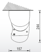
Pose plafond maxi 90°
