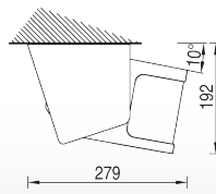
Pose plafond Inclinaison de 5° à 75°
