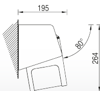
Pose de face Inclinaison de 10° à 90°
