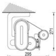
Pose plafond Inclinaison de 5° à 75°
