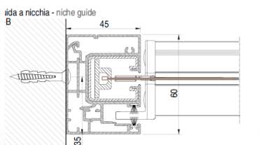
Pose en niche
