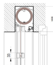
Barre de charge 33x45 Coffre 110 x155
