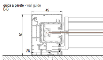
Pose de face
