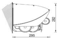
Pose de face Inclinaison de 5° à 75° (10° si avancée < 3600 mm)
