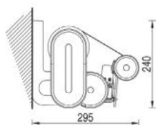
Pose de face Inclinaison de 5° à 75° (10° si avancée < 3600 mm)
