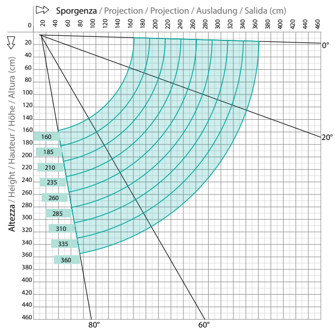
Diagramm für Wandbefestigung
