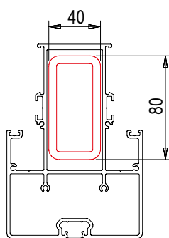
Träger aus verstärktem Glas
