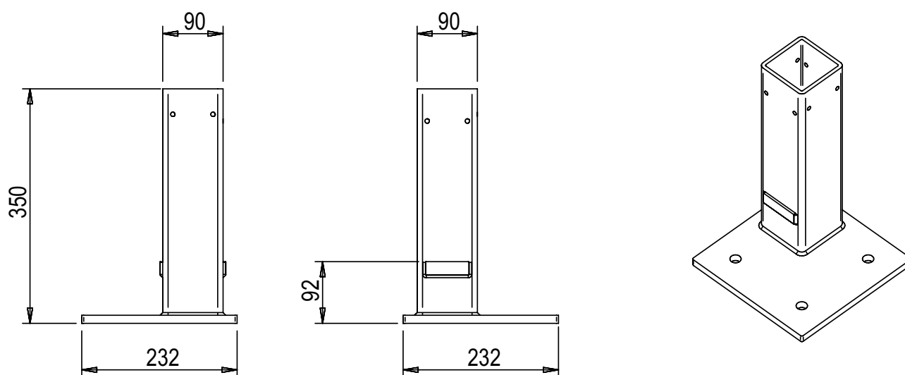
OPTIONAL - Fuß mit außenliegender Basis
