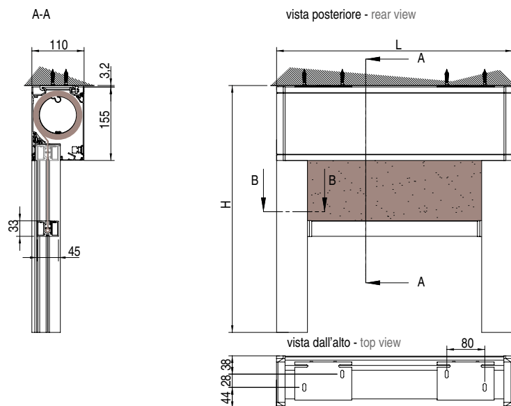
guida a nicchia - niche guide
