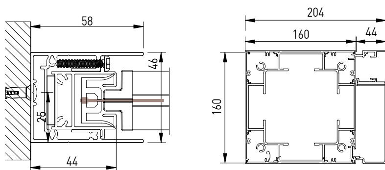
Guide sur les colonnes/mur
