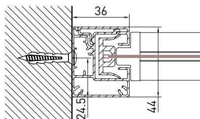
Nischenführung B-B
