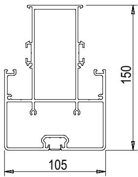
Poutre standard pour porte vitrée
