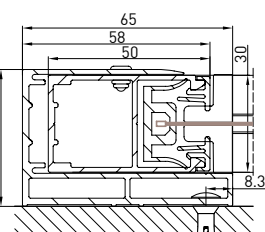
Guida a parete (GCP)
