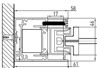
B-B
