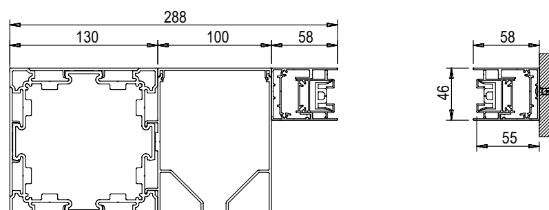
Fissaggio colonna con scarico - parete
