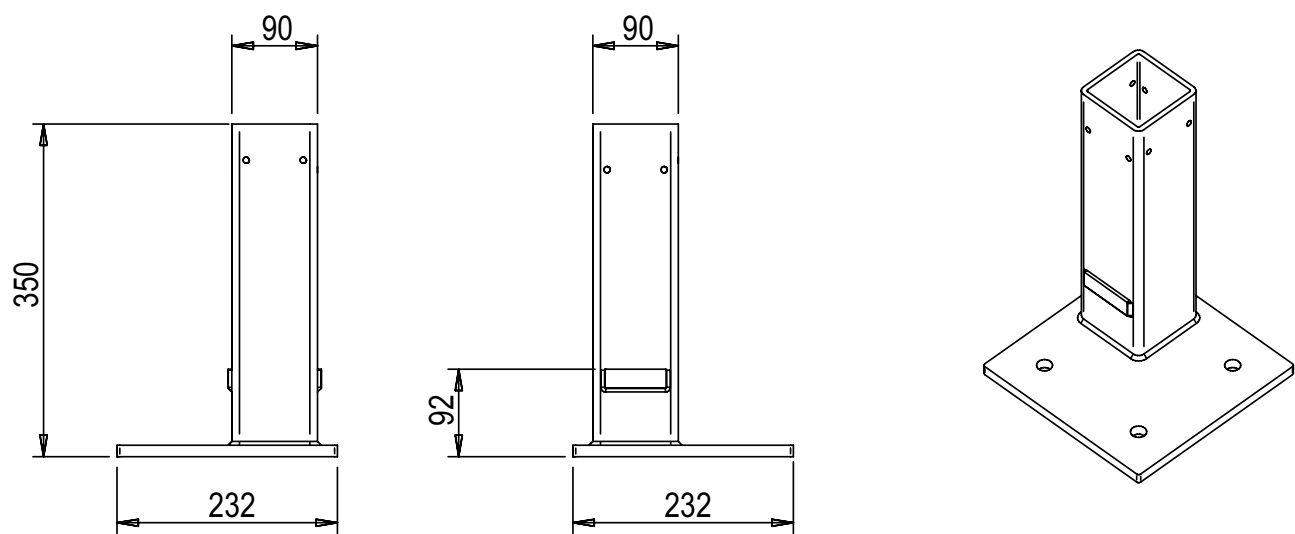
OPTIONAL - Piedino con base esterna
