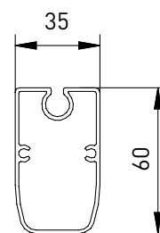
Traverse porte-tissu
