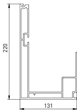
Gouttière
