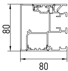
Führungsschiene
