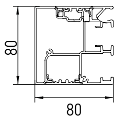
Führungsschiene
