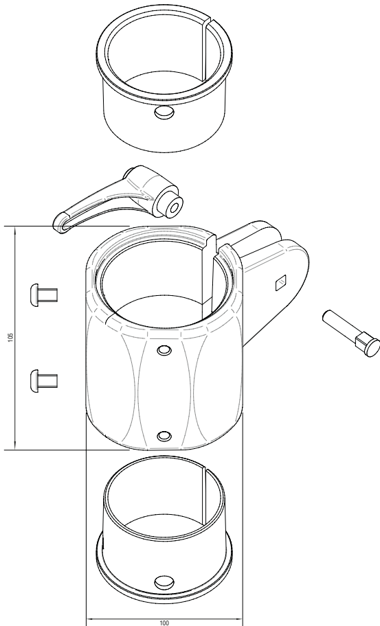
Elemento corredizo para árbol
