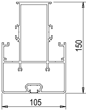
Viga frontal
