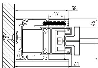
Nischenführung B-B
