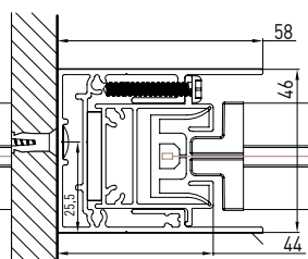
Guida a nicchia B-B
