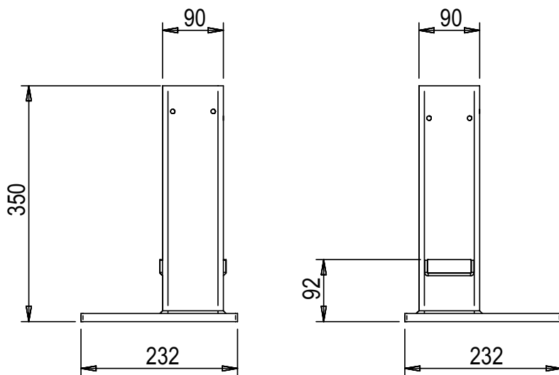
OPTIONAL - Piedino con base esterna
