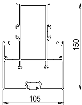
Barre frontale
