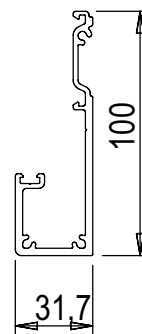
Seitlicher Glasträger
