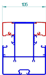
Profil A
