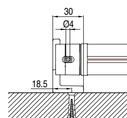
Nischenbefestigung B-B
