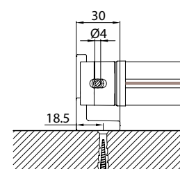
Nischenbefestigung B-B
