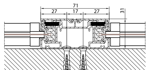
Guida a parete (modulo doppio) C-C
