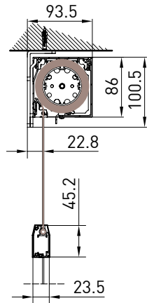
QUADRO - SQUARE A-A
