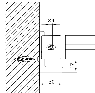
piedino a pavimento - floor bracket B-B
