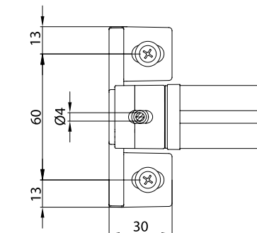
piedino a pavimento - floor bracket B-B
