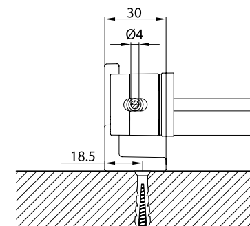
supporto a nicchia - niche bracket B-B
