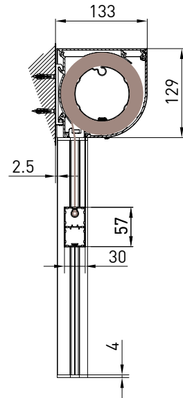
TONDO - ROUND A-A
