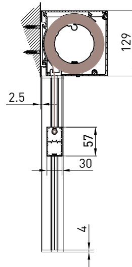
QUADRO - SQUARE A-A
