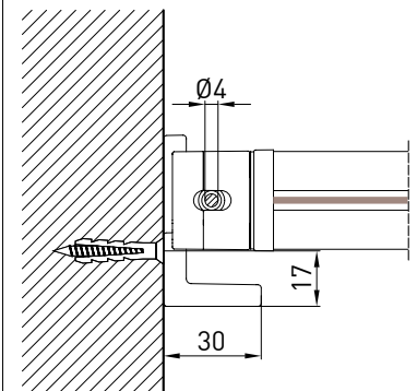
pedino a pavimento - floor bracket B-B
