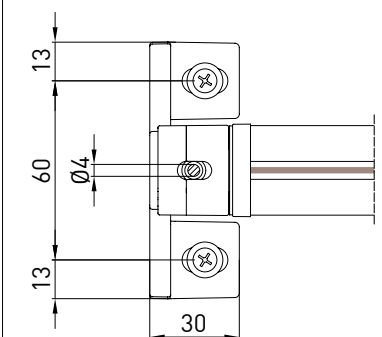
pedino a pavimento - floor bracket B-B
