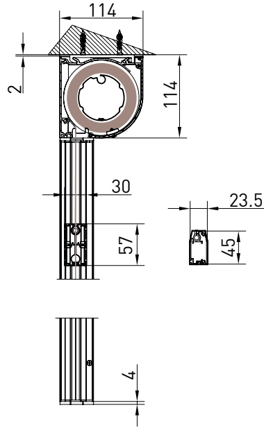
TONDO - ROUND A-A
