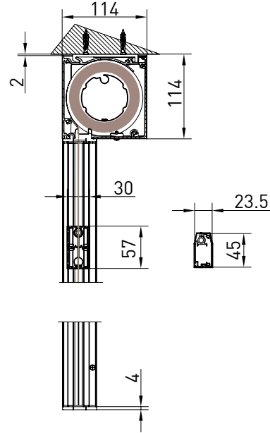
QUADRO - SQUARE A-A
