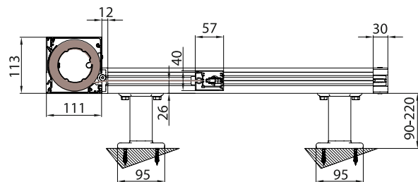
QUADRO - SQUARE A-A
