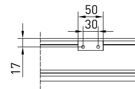
B-B
