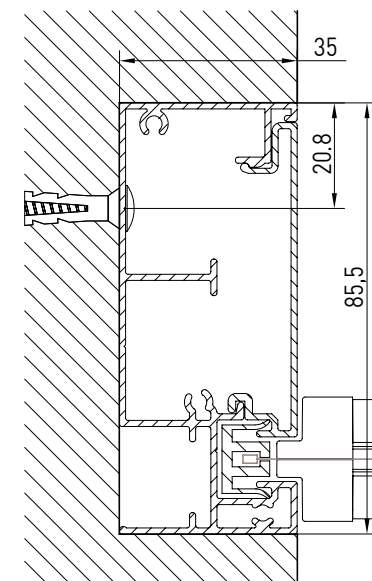
B-B
