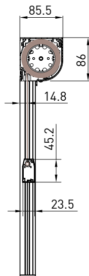
TONDO - ROUND A-A
