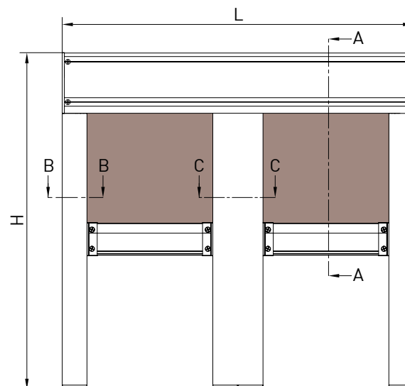
vista posteriore - rear view cassonetto unico - single cassette
