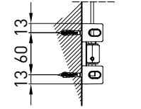
Piedino a pavimento - Floor foot - Pied sol - Bodenbefestigung
