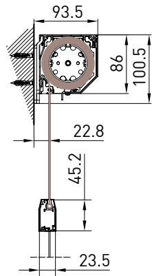
SMUSSATO - BEVELLED A-A
