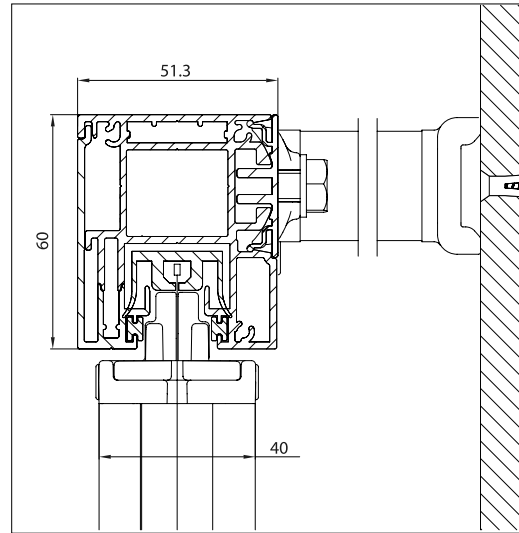
guida a parete - wall guide B-B
