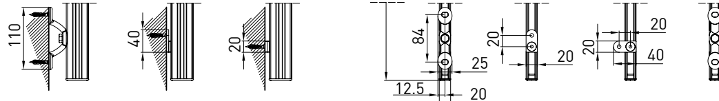
Guida a nicchia - Niche guide - Coulisse tableau - Nischenführung
