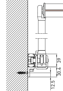
guida a nicchia - niche guide B-B
