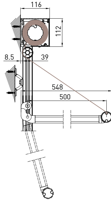
QUADRO - SQUARE A-A
