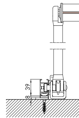
guida a parete - wall guide B-B
