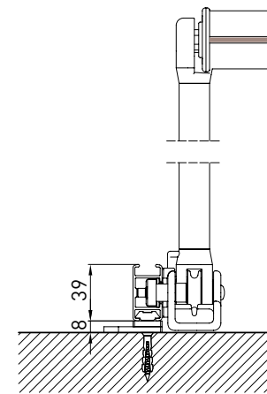
guida a parete - wall guide B-B
