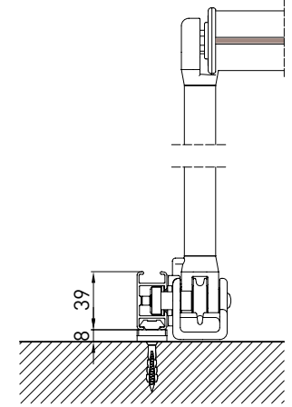
guida a parete - wall guide B-B
