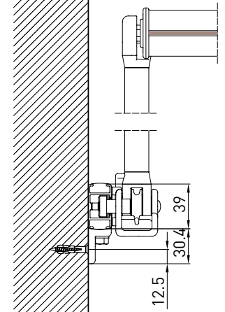
guida a nicchia - niche guide B-B
