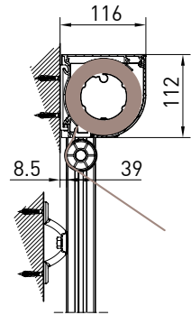
TONDO - ROUND A-A
