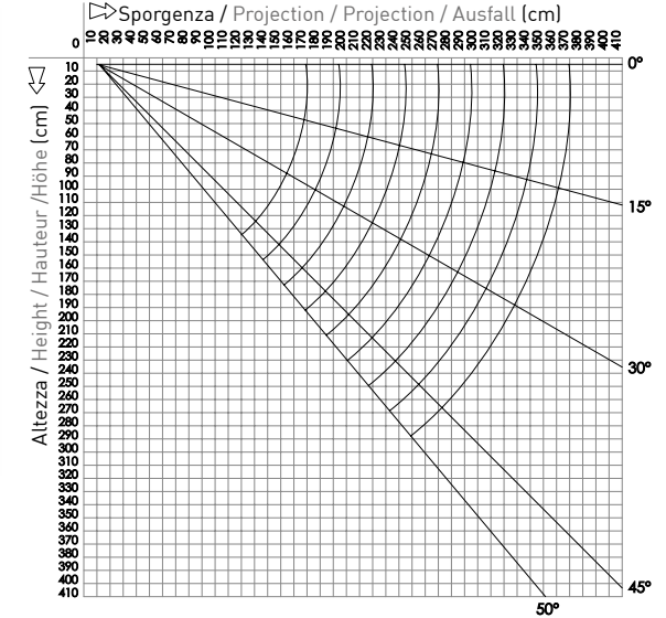
Diagramma di copertura a parete/soffitto - Wall/Ceiling Covering diagram
